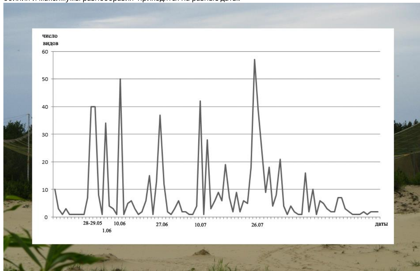
Рис. 1. Динамика видового состава жесткокрылых, привлеченных светом в 2018 году.
