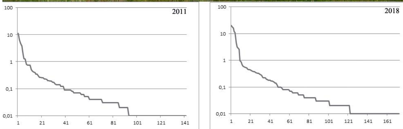
Рис. 2. Кривые доминирования-разнообразия для Coleoptera из светоловушки 2011 и 2018 гг.
