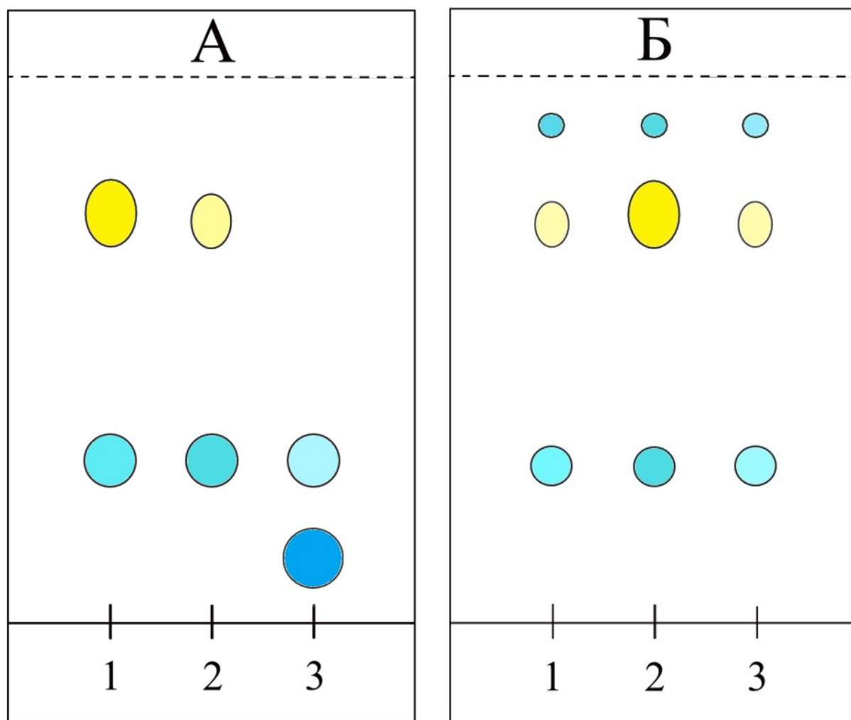
Схема ТСХ хроматограмм водно-спиртовых извлечений из сырья видов рода Боярышник: А – почки; Б – кора. Обозначения: 1 – боярышник кроваво-красный; 2 – боярышник вееровидный; 3 – боярышник мягковатый
