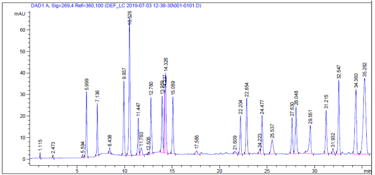
Рис. 1. Хроматограмма стандартной смеси аминокислот
