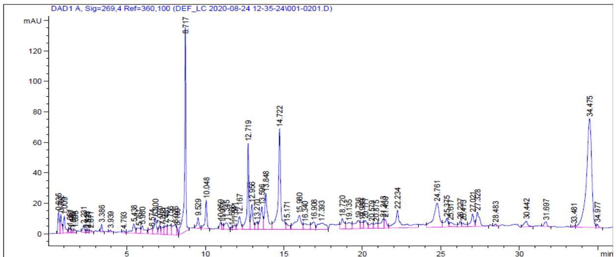
Рис. 2. Хроматограмма сухого экстракта «Фитоинфлам»
