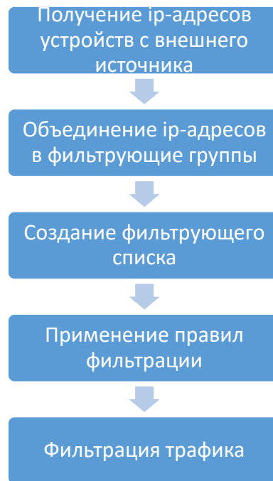
Рисунок 2. Алгоритм работы программного обеспечения.
