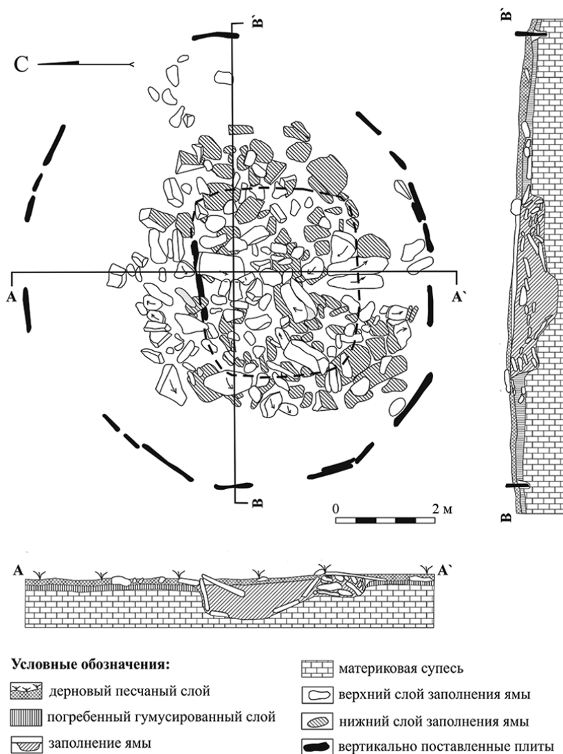
Рис. 5. Объект №51 комплекса Нижняя Соору. План и разрез
