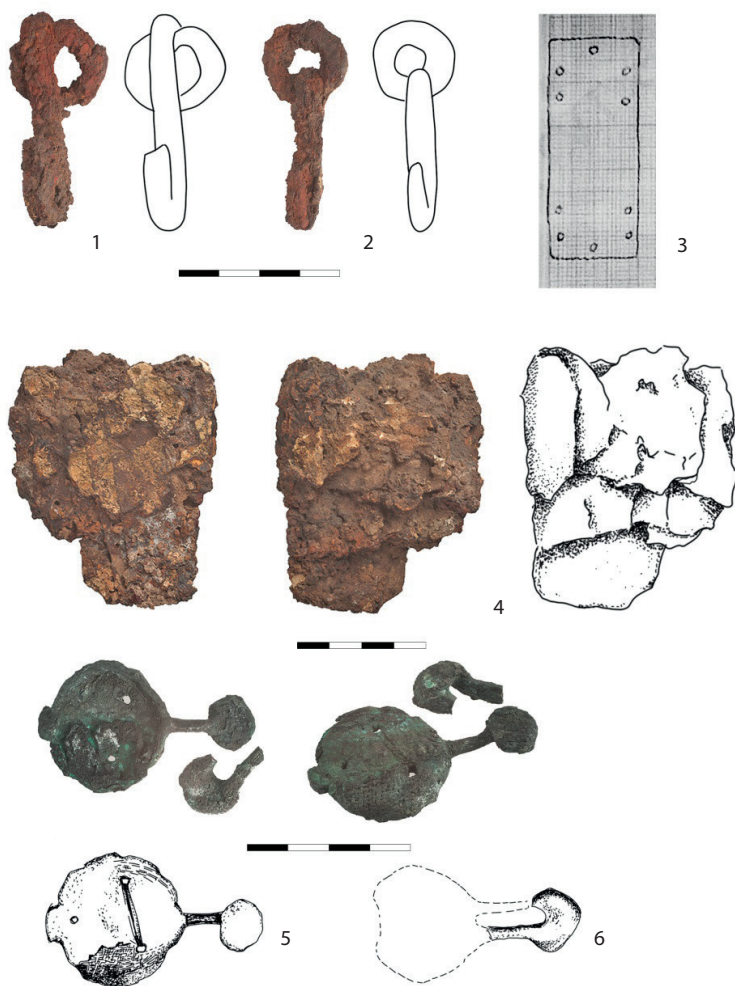
Рис. 2. БКМ. Курган №1, погребение 3: 1, 2 – железные крюки; 3 – панцирная пластина; 4 – спекшиеся панцирные пластины; 5 – бронзовая двусоставная застежка; 6 – часть бронзовой двусоставной застежки. 3 – по: (Дульзон, Научный архив, с. 125), 6 – по: (Дульзон, 1947а, табл. 33, №16)
