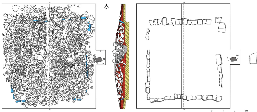
Рис. 4. План и разрез ограды № 1 комплекса Устийн ам Fig. 4. Plan and section of fence No. 1 of the Ustiin am
