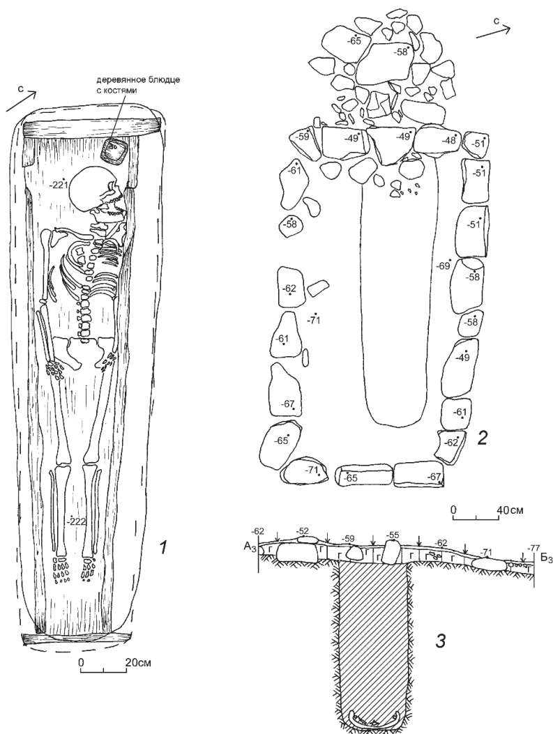
Рис. 7. План кургана 41. 1 – план погребения; 2 – план крепиды, 3 – профиль объекта Fig. 7. Plan of barrow 41. 1 – burial; 2 – stone base of barrow, 3 – profile of barrow
