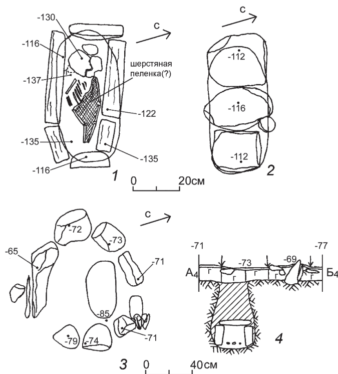
Рис. 8. План кургана 41а. 1 – план погребения; 2 – план перекрытия; 3 – план крепиды; 4 – профиль объекта
