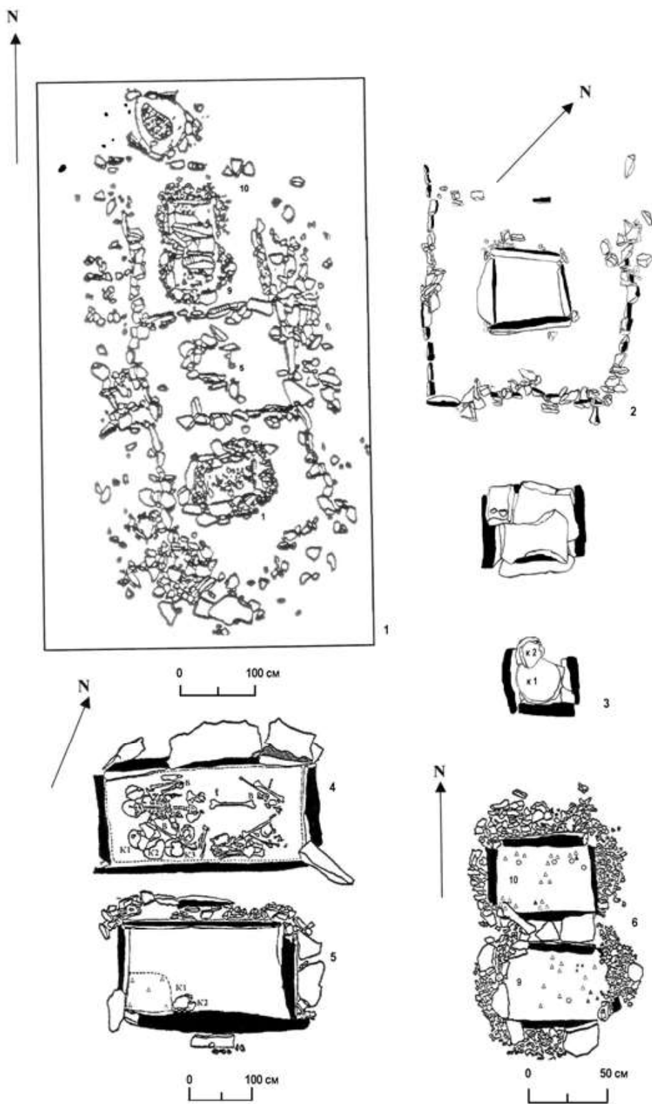
Рис. 3. Погребальные конструкции комплекса Ой-Джайляу: 1, 6 - могильник Ой-Джайляу-VII; 2, 3 - могильник Ой-Джайляу-IX; 4, 5 - могильник Ой-Джайляу-III.
