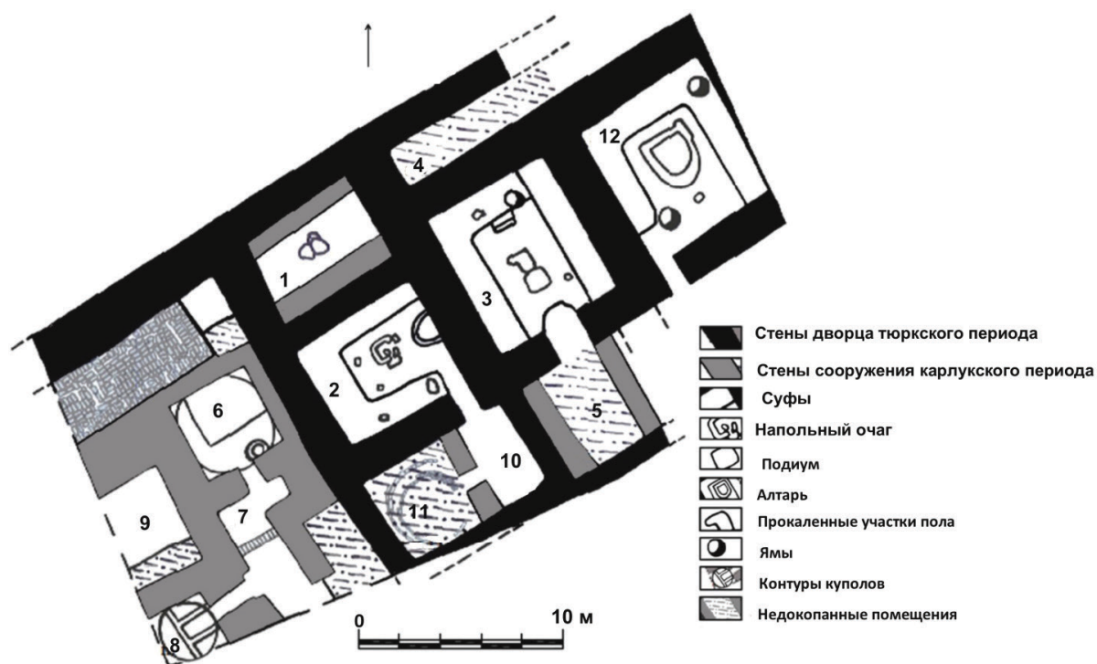
Рис. 1. План раскопанной части цитадели городища Луговое
