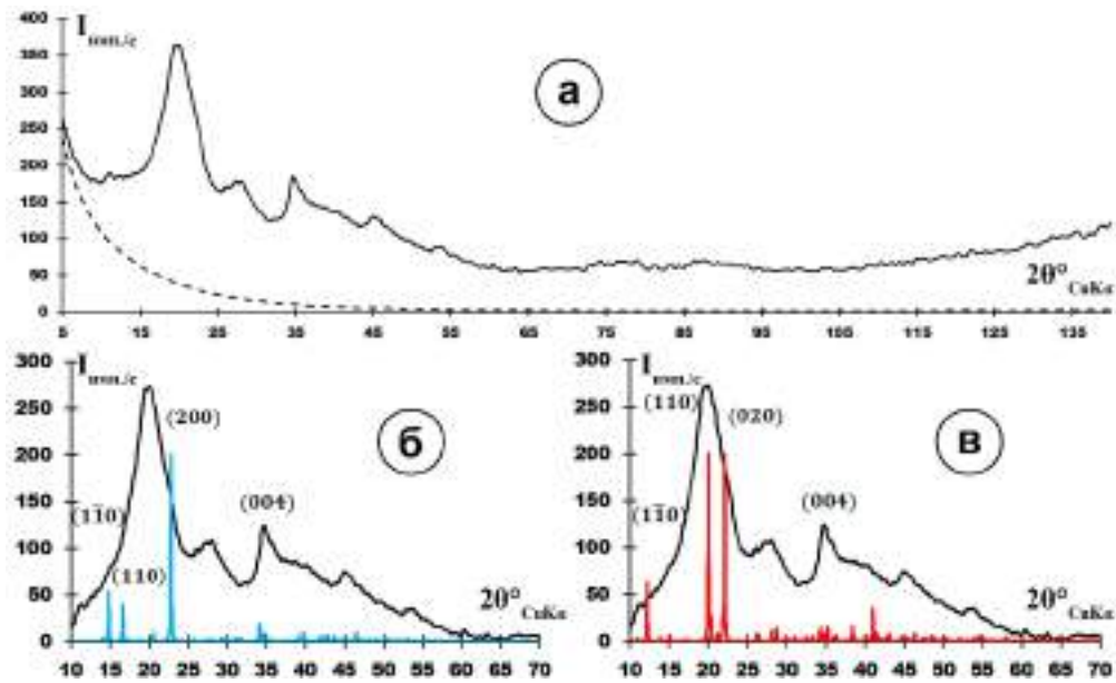
Рис. 2. Рентгенограммы исследуемого образца ПЦ — и воздуха — — (а) в сравнении с теоретическими рентгенограммами, построенные для фаз целлюлозы I \beta — (рис. 2б) и целлюлозы II — (рис.2в).
