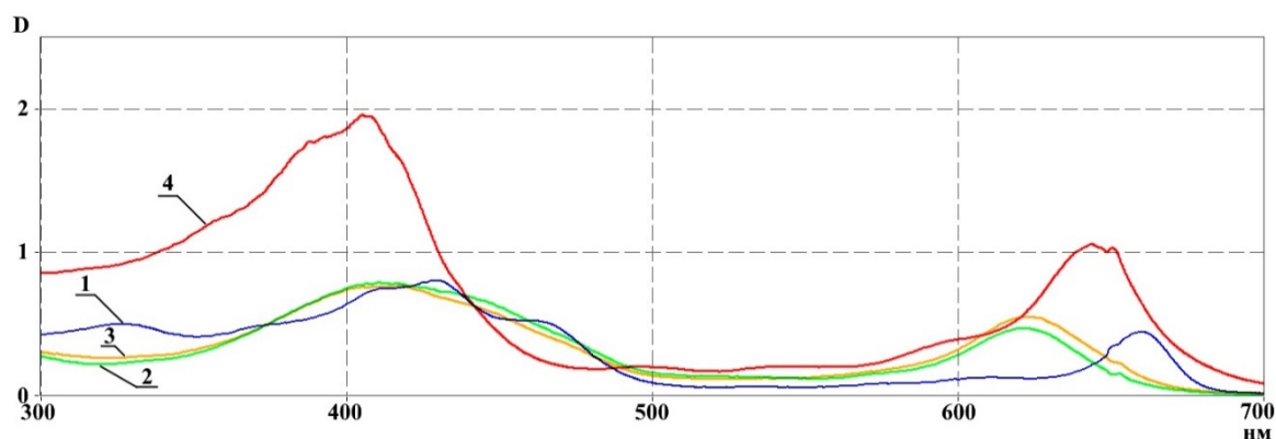
Рис. 1. Спектры поглощения в ультрафиолетовой и видимой области следующих образцов: 1 – извлечение из листьев крапивы двудомной; 2 – «Хлорофилл питьевой травяной»; 3 – заводской экстракт крапивы; 4 – фракция медного комплекса хлорофилла, полученная при делении заводского экстракта
