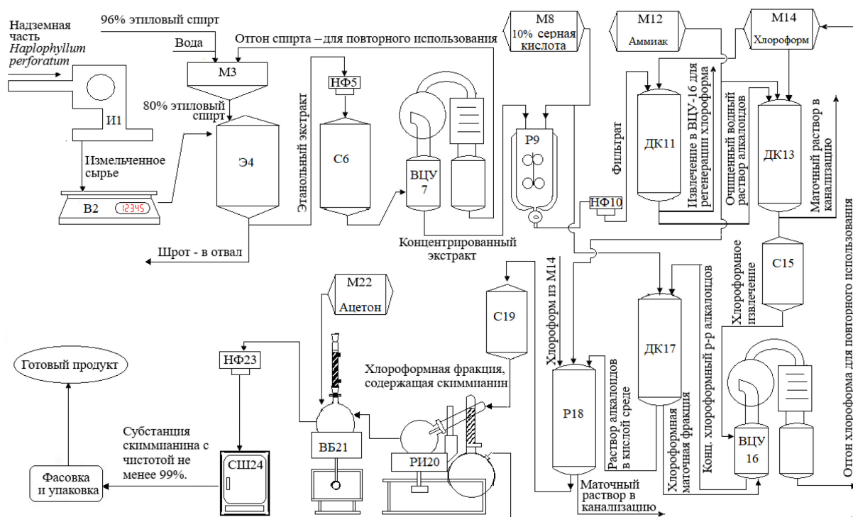
Рис. 3. Аппаратурная схема производства скиммианина из н/ч цельнолиственного исколотого И1 – мельница; В2 – весы; М3, М8, М12, М14, М22 – мерники; Э4 – экстрактор; НФ5, НФ10, НФ23 – нутч-фильтры; С6, С15, С19 – сборники; ВЦУ7, ВЦУ16 – вакуум-циркуляционные выпарные аппараты; Р9, Р18 – реакторы; ДК11, ДК13, ДК17 – делительные колонки; РИ20 – ротационный испаритель; ВБ21 – водяная баня; СШ24 – сушильный шкаф
