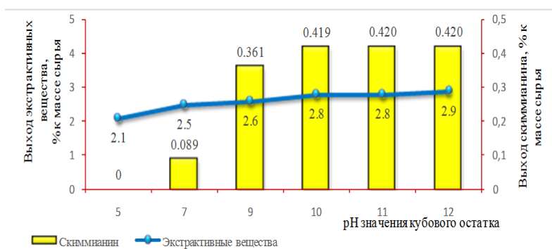
Рис. 1. Влияние pH кубового остатка на выход скиммианина при экстракции хлороформом
