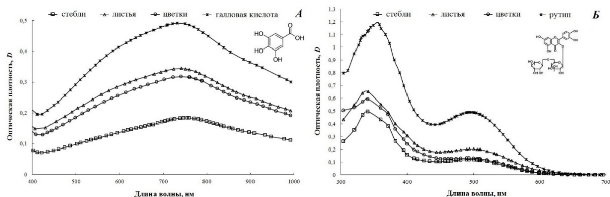
Рис. 1. Спектры светопоглощения комплексов, образованных: А – реактивом ФЧ с фенольными соединениями, содержащимися в экстрактах Б из стеблей, листьев и цветков D. fruticosa (ЦП 3) и с раствором ГК концентрацией 0.01 г/100 мл; Б – 5%-ным раствором \text{AlCl}_3 с флавоноидами, содержащимися в экстрактах Б из стеблей, листьев и цветков D. fruticosa (ЦП 1) и с раствором рутина концентрацией 1000 мкг/мл
