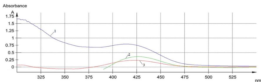
Рис. 1. УФ-спектр комплекса флавоноидов шрота корня солодки с \text{AlCl}_3 : 1 – без добавок, 2 – с ацетатом натрия, 3 – с уксусной кислотой
