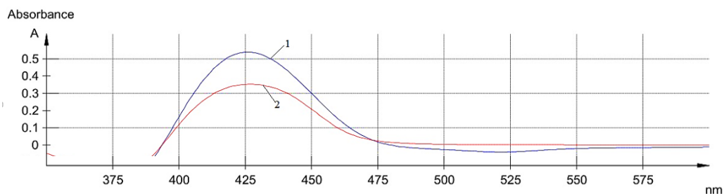
Рис. 2. 1 – УФ-спектр комплекса флавоноидов экстракта шрота корня солодки с \text{AlCl}_3 (в присутствии ацетата натрия), 2 – УФ-спектр комплекса кверцетина с \text{AlCl}_3
