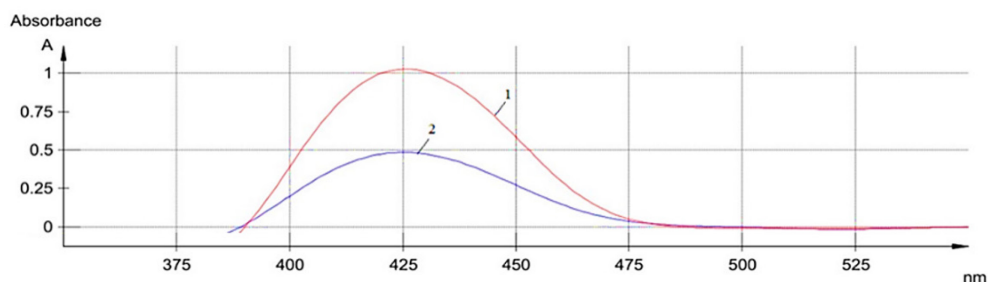
Рис. 3. УФ-спектры комплексов флавоноидов с \text{AlCl}_3 в экстрактах корня (1) и шрота (2) солодки, полученных 70% этанолом
