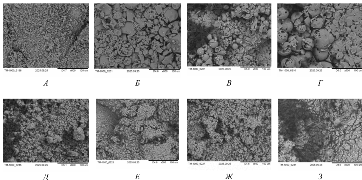
Рис. 1. Электронные микрофотографии исходных веществ и полученных твердых дисперсий. Масштабы приведены на фотографиях. А – КВ, Б – АГ, В – \text{Na}_2\text{ГК} , Г – ГП-ЦД, Д – ТД КВ с АГ (1/10 вес.), Е – ТД КВ с \text{Na}_2\text{ГК} (1/10 вес.), Ж – ТД КВ с ГП-ЦД (1/1 мол.), З – ТД КВ с ГП-ЦД (1/2 мол.)
