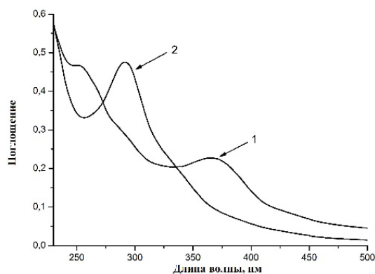
Рис. 5. УФ-спектр продукта окисления KB ионами \text{Fe}^{3+} в системе с чистым KB. Спектр 1 – нулевая точка, спектр 2 – через 1 ч после начала реакции при комнатной температуре
