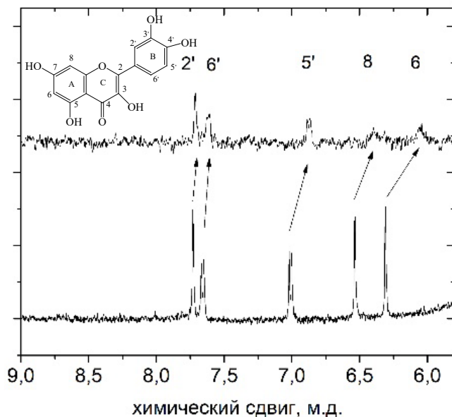
Рис. 2. Фрагменты спектров ^1\text{H} ЯМР ароматических протонов кверцетина в 50% растворе \text{CD}_3\text{OD} в \text{D}_2\text{O} (внизу) и комплекса кверцетина с ГП-ЦД в \text{D}_2\text{O} (вверху) при температуре 30^\circ\text{C} . Нумерация протонов КВ указана на структурной формуле
