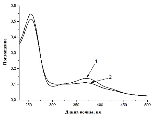
Рис. 7. УФ-спектр продукта окисления KB ионами \text{Fe}^{3+} в системе с механохимически полученным комплексом KB с \text{Na}_2\text{ГК} . Спектр 1 – нулевая точка, спектр 2 – через 1 час после начала реакции
