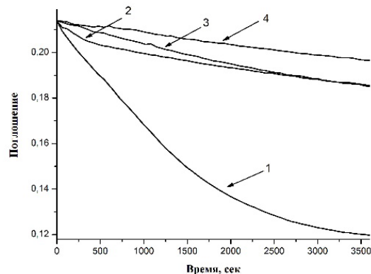
Рис. 8. Изменение поглощения от времени на длине волны 361 нм в реакции окисления KB ионами \text{Fe}^{3+} . Кривая 1 – в системе с чистым KB, в системе с механохимически полученным комплексом – кривая 2 – KB с \text{Na}_2\text{ГК} , 3 – KB с ГП-ЦД (1/2 мол.), 4 – KB с ГП-ЦД (1/1 мол.)
