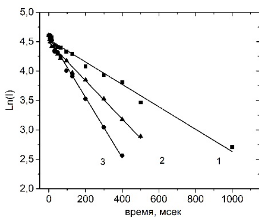
Рис. 3. Зависимости интенсивности сигнала эха в эксперименте СРМГ (в логарифмическом масштабе) ароматических протонов 2'-Н КВ от времени в водно-метанольном растворе при температуре 30^\circ\text{C} . (1) КВ; (2) КВ-АГ; (3) КВ- \text{Na}_2\text{ГК} . Точки – эксперимент, сплошные линии – расчет. Расчетные времена релаксации приведены в тексте. Погрешность расчета не превышает 5%
