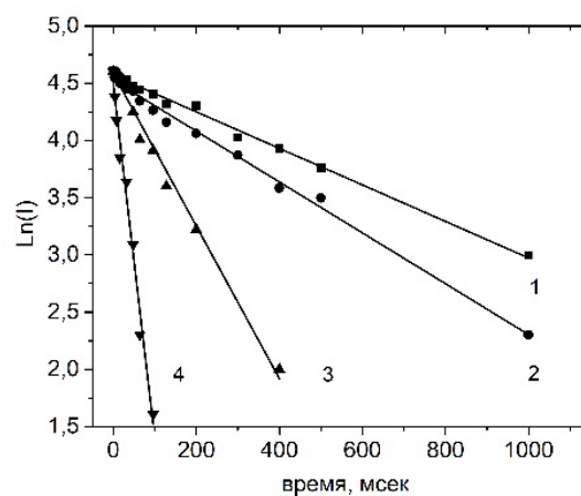
Рис. 4. Зависимости интенсивности сигнала эха в эксперименте СРМГ (в логарифмическом масштабе) ароматических протонов 8-Н и 5'-Н КВ в водно-метанольном растворе, и КВ-ГП-ЦД (1 : 2) от времени в водном растворе при температуре 30^\circ\text{C} . (1) 5'-Н КВ; (2) 8-Н КВ; (3) 5'-Н КВ-ГП-ЦД; (4) 8-Н КВ-ГП-ЦД. Точки – эксперимент, сплошные линии – расчет. Расчетные времена релаксации приведены в тексте. Погрешность расчета не превышает 5%
