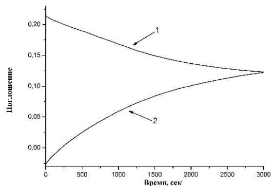
Рис. 6. Изменение поглощения KB на длине волны 361 нм – кривая 1 и продукта окисления KB ионами \text{Fe}^{3+} на длине волны 291 нм – кривая 2 в системе с чистым KB
