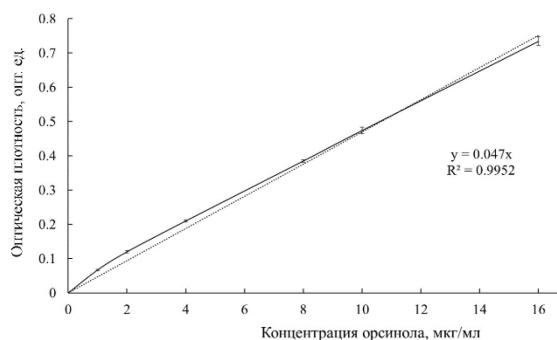
Рис. 5. Калибровочная кривая для определения содержания АР. Пунктирной линией отмечена линия тренда для калибровочной кривой. Коэффициент корреляции и уравнение регрессии представлены на рисунке
