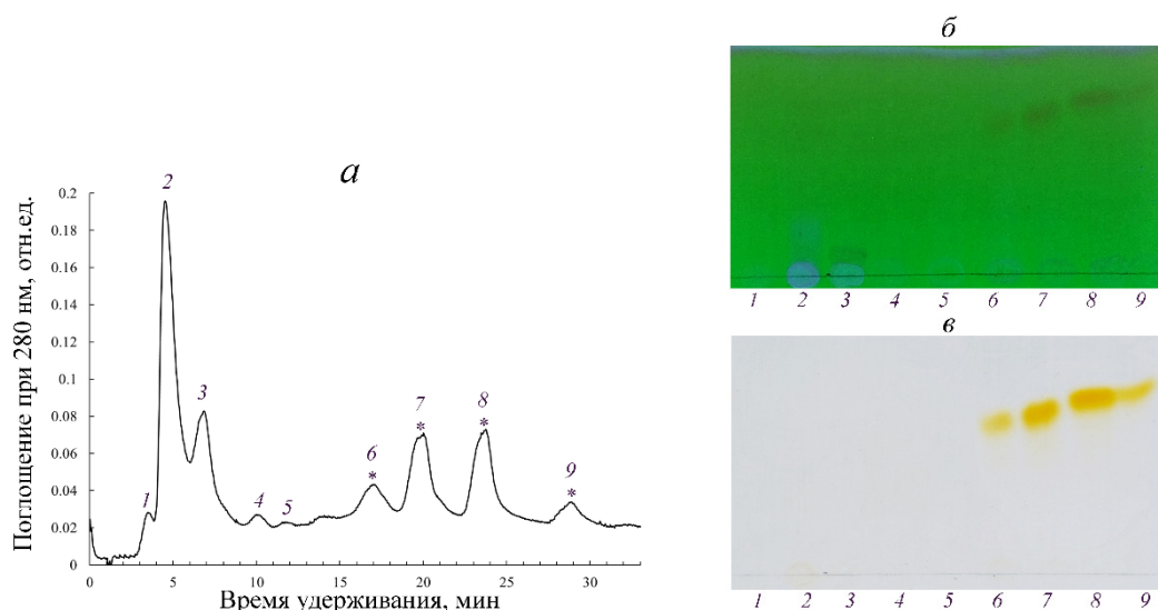
Рис. 3. ВЭЖХ экстракта из ЦЗМ мягкой яровой пшеницы сорта Ситара (а) и ТСХ-анализ (б, в) фракций, собранных при проведении ВЭЖХ (пики 1–9): флуоресценция при 312 нм (б), качественная реакция на резорциновые липиды (в). 1–9 – фракции с 1 по 9. Звездочками на хроматограмме (а) отмечены фракции, прореагировавшие положительно (в)
