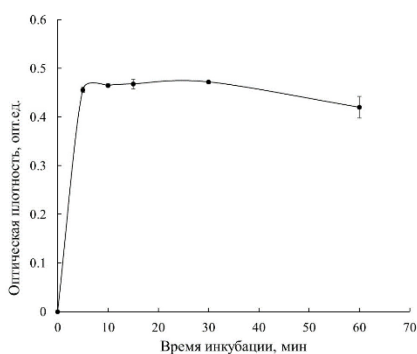
Рис. 4. Значения оптической плотности продукта реакции орсинола (10 мкг/мл) с солью Fast Blue RR при 483 нм через 5, 10, 15, 30 и 60 мин после смешивания компонентов реакционной смеси
