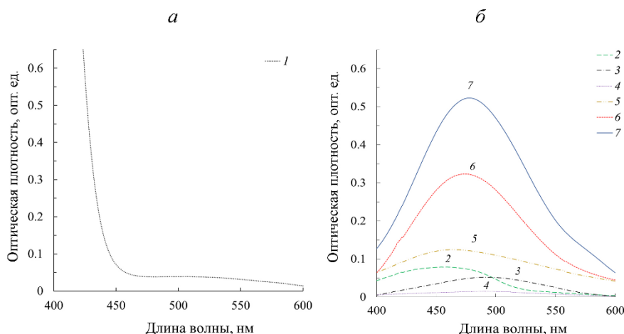
Рис. 1. Спектры поглощения диазониевой соли Fast Blue RR (а) и продуктов реакции фенольных соединений (80.6 мкМ) с солью Fast Blue RR (б). 1 – Fast Blue RR, 2 – феруловая кислота, 3 – галловая кислота, 4 – апигенин, 5 – кверцетин, 6 – катехин, 7 – орсинол
