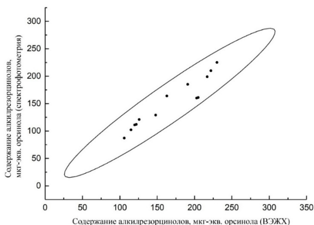
Рис. 6. Корреляция между данными по содержанию АР в ЦЗМ мягкой яровой пшеницы, полученными методом ВЭЖХ (ось абсцисс) и спектрофотометрическим методом (ось ординат)
