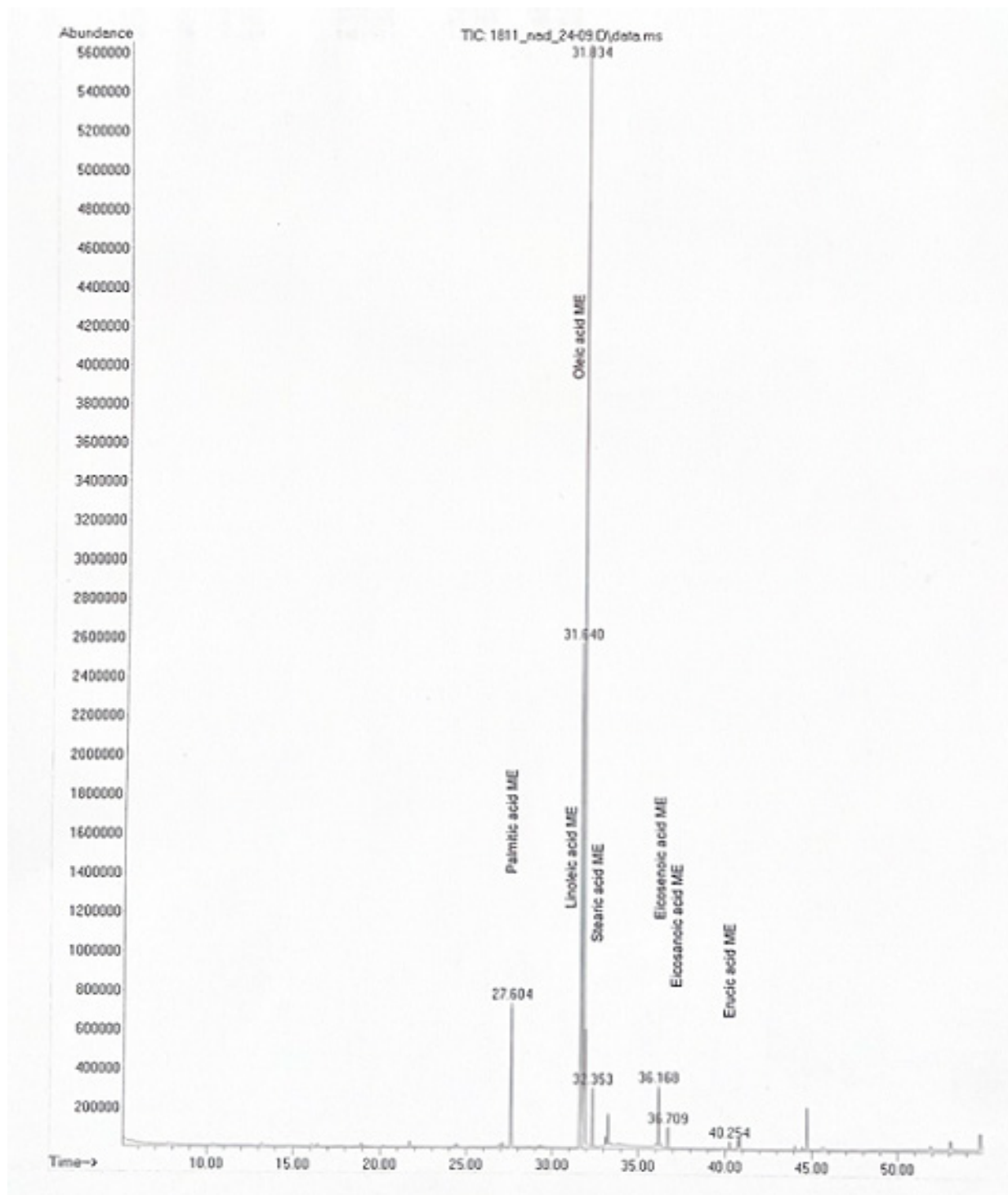
Газохроматографическое разделение метиловых эфиров кислот рапсового масла
