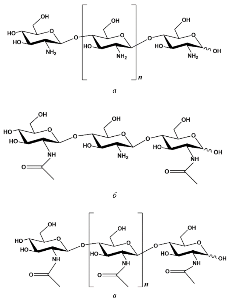
Рис. 1. Типы хитоолигосахаридов: а) полностью деацетилированные; б) частично ацетилированные; в) полностью ацетилированные [10]
